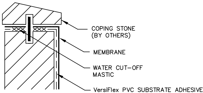
VersiFlex VFC-9E COPING STONE TERMINATION
