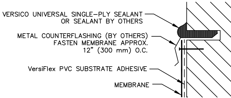
VersiFlex VFC-9C COUNTERFLASHING TERMINATION
